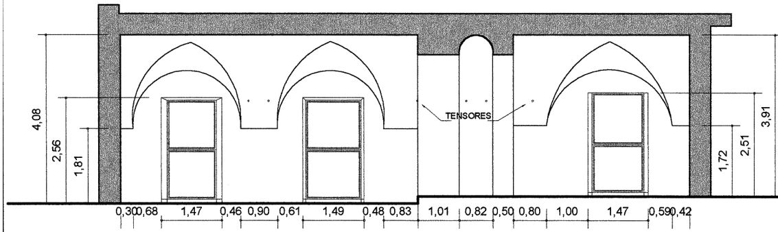
CORTE A-A
