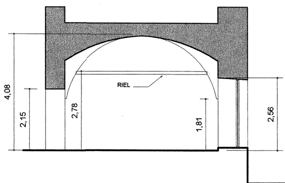
CORTE C-C
