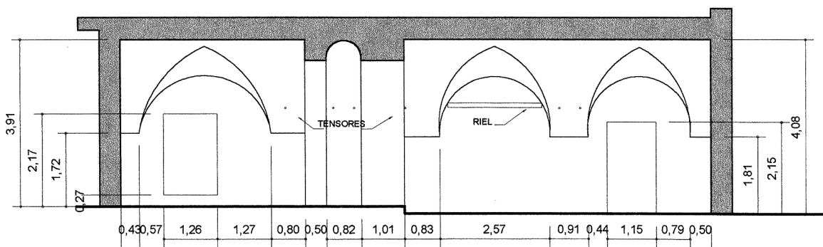
CORTE D-D
